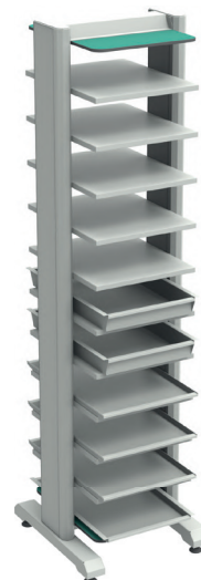
СТЕЛЛАЖ ДЛЯ СПЕЦ. ЛОТКОВ СТЛ-3А
